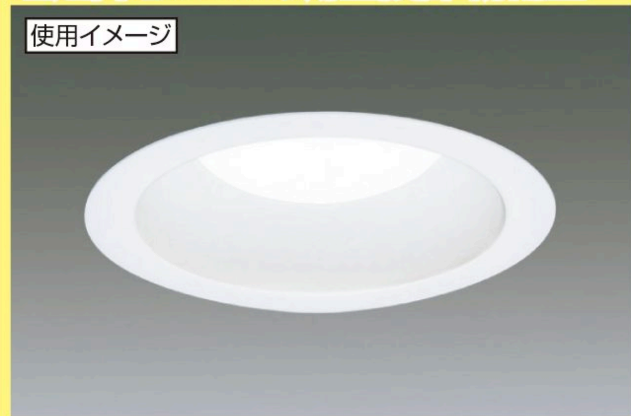
LEDダウンライト (LSB100-0650NCAW-V3) 昼白色 (LSB100-0627NCAW-V3) 電球色 埋込穴φ100
